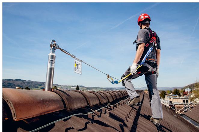
Fig. 5: Classe d'équipement 2; ligne de vie
